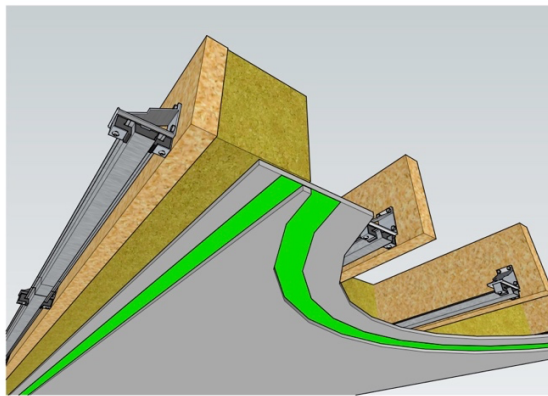
Figur 20: Metallholder for å bygge klipsen inn i trebjelkelag uten å måtte kubbe på tvers.
