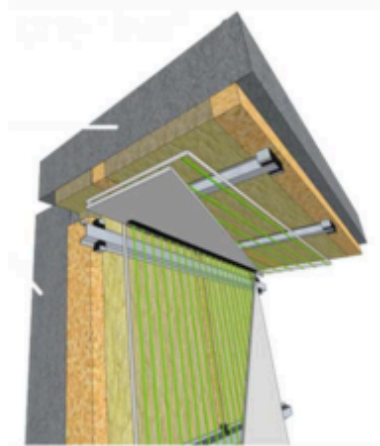
Figur 2. Illustrasjon av lydisolert vegg og himling ved hjelp av gummiavkobling. Figur er hentet fra https://dreamscreen.no .
