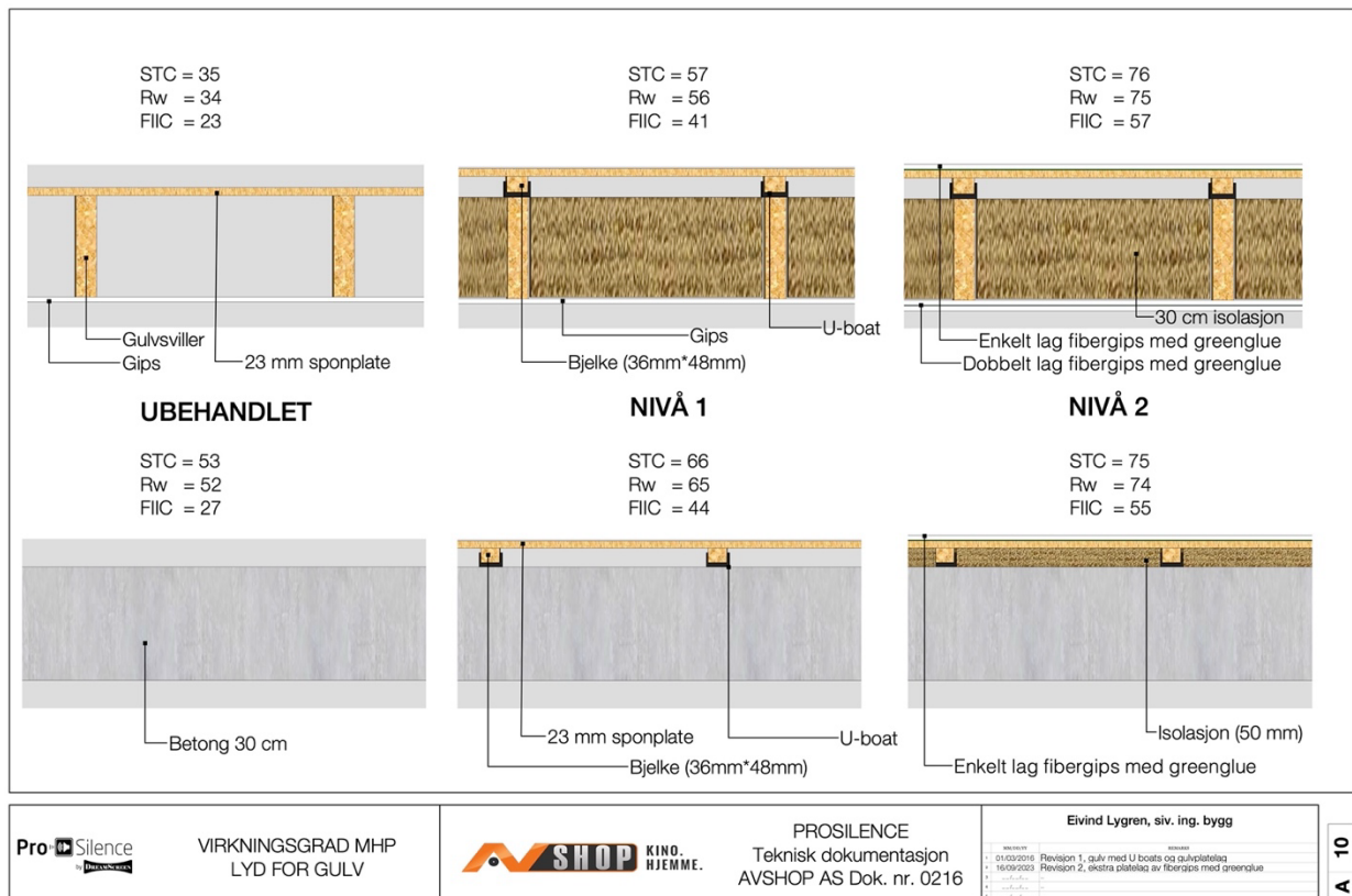
Figur 13: STC, Rw og FIIC for gulv. Ubehandlet og nivå 1 og 2 med Prosilence.
