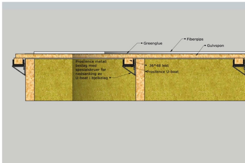
Figur 12: Metallholder for å forsænke U boat i trebjelkelag og evt avrette gulvbjelkelag.
